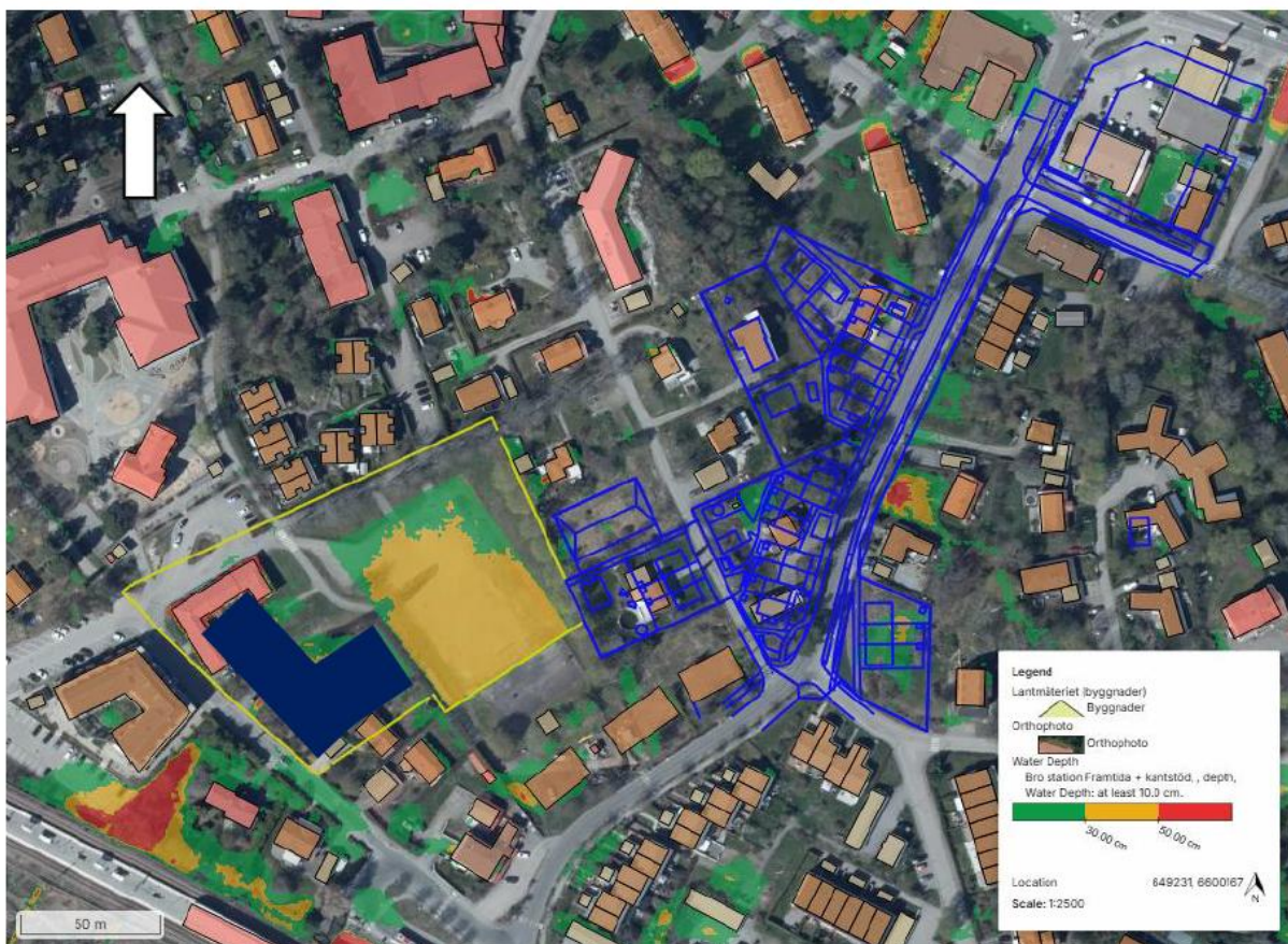
Figur 28 Illustration från dagvattenutredning för Nya Härneviskolan som visar hur vatten samlas på nedsänkt bollplan, med ca 30-50 cm djup. Planområdet för Norra Köpmanvägen illustreras med blå linjer, Härneviskolan med fylld blå polygon.
