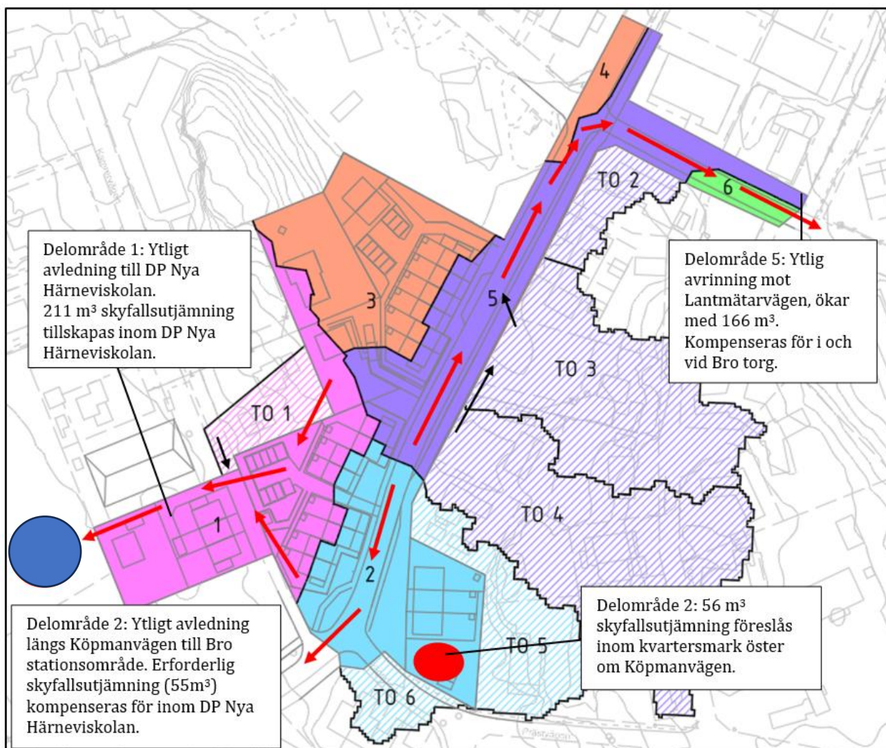
Figur 30. Flödesriktningar efter exploatering samt principiellt förslag till placering av översvämningsytor inom planområdet (röd yta). Kompletterande yta utom planområdet redovisas med blå cirkel. Bild Marktema, justerat avseende delområde 5.
