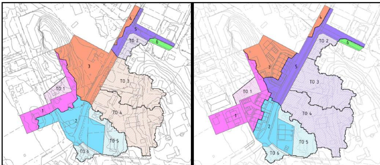
Figur 31. Jämförelse mellan topografiska delavrinningsområden, befintligt till vänster och planerat till höger. Av bilden framgår att område 3 minskar och att tillrinningsområde 4 avleds till område 5 istället för till område 3. Bild: Marktema
