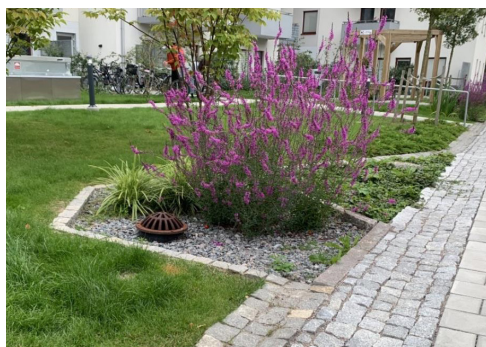
Nedsänkt växtbädd på gemensam gårdsyta.
